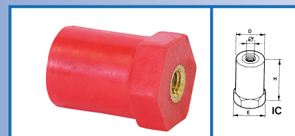
Isolatoren Serie IC Insulators Series IC
