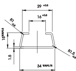
Profil 3415
