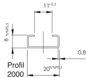
Profil 2000 Auch mit Lochung lieferbar
