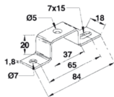
Abstandhalter
