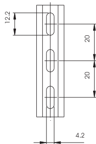
Lochung für Profil 1555
