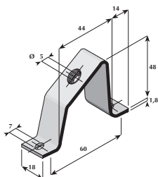
Schrägmontagewinkel
