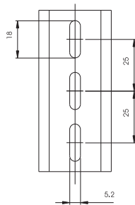
Lochung für Profil 3575, 3515 und 3215
