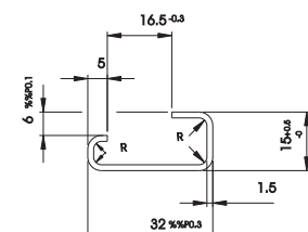
Profil 3215
