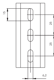
Sonderlochung für Profil 3575 und 3515
