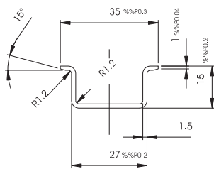
Profil 3515
