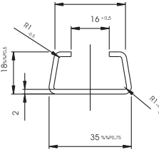
Profil 3518 Auch mit Lochung lieferbar
