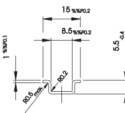
Profil 1555
