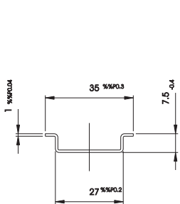
Profil 3575
